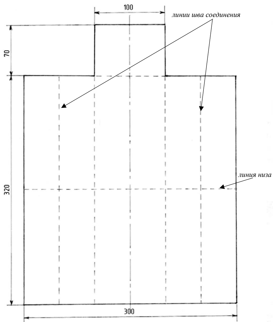
Рисунок 2. Чертеж конструкции чехла
