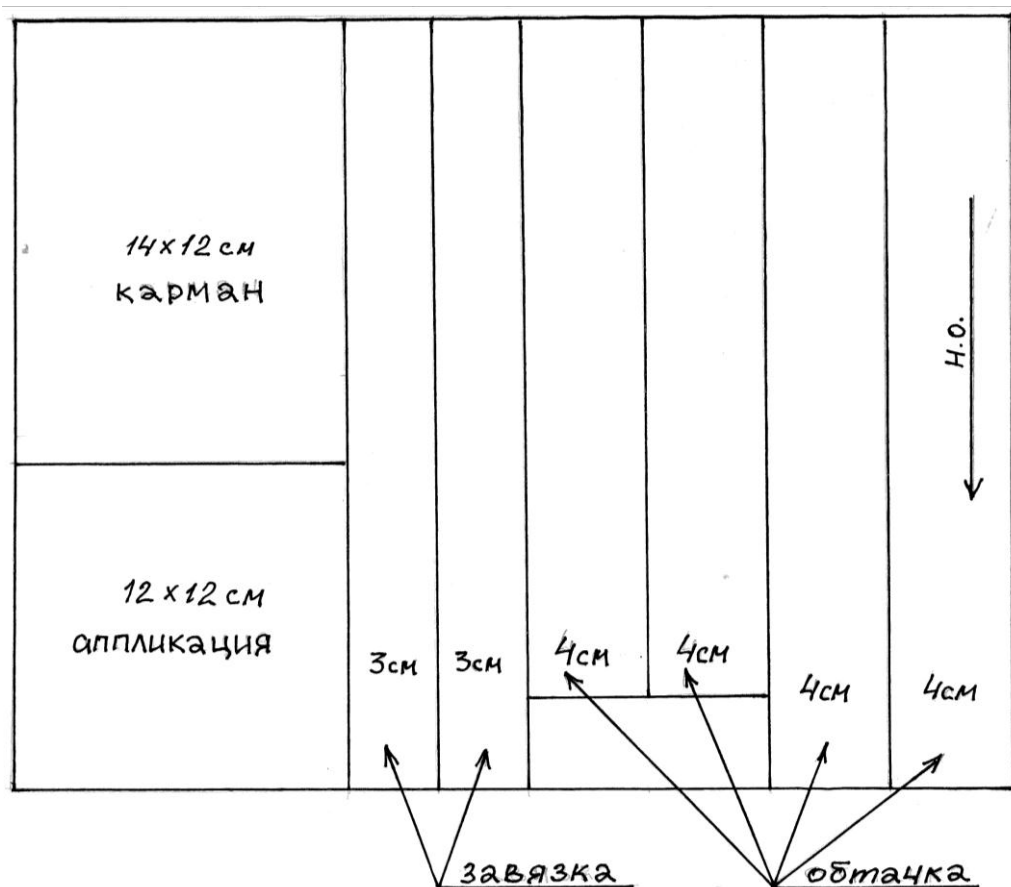
Рисунок 2. Раскладка деталей из отделочной ткани
